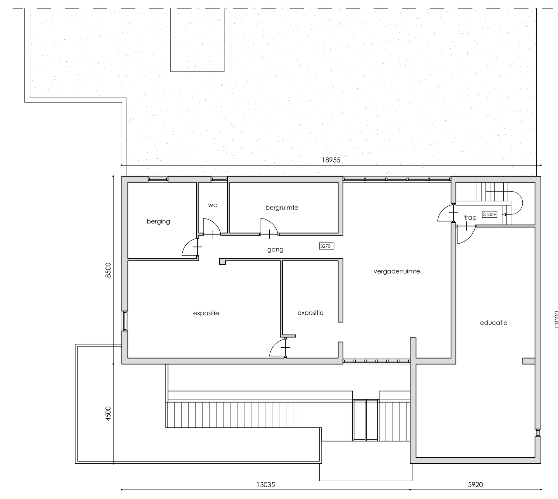
VERDIEPING BESTAAND
