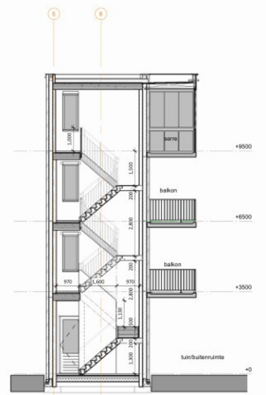
Doorsnede D
