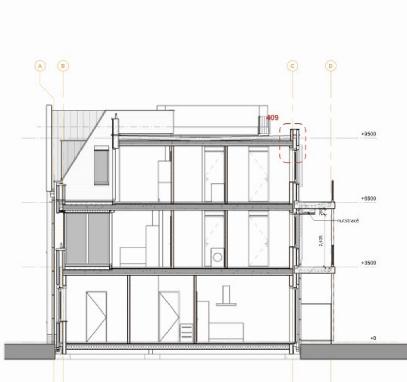
Doorsnede E
