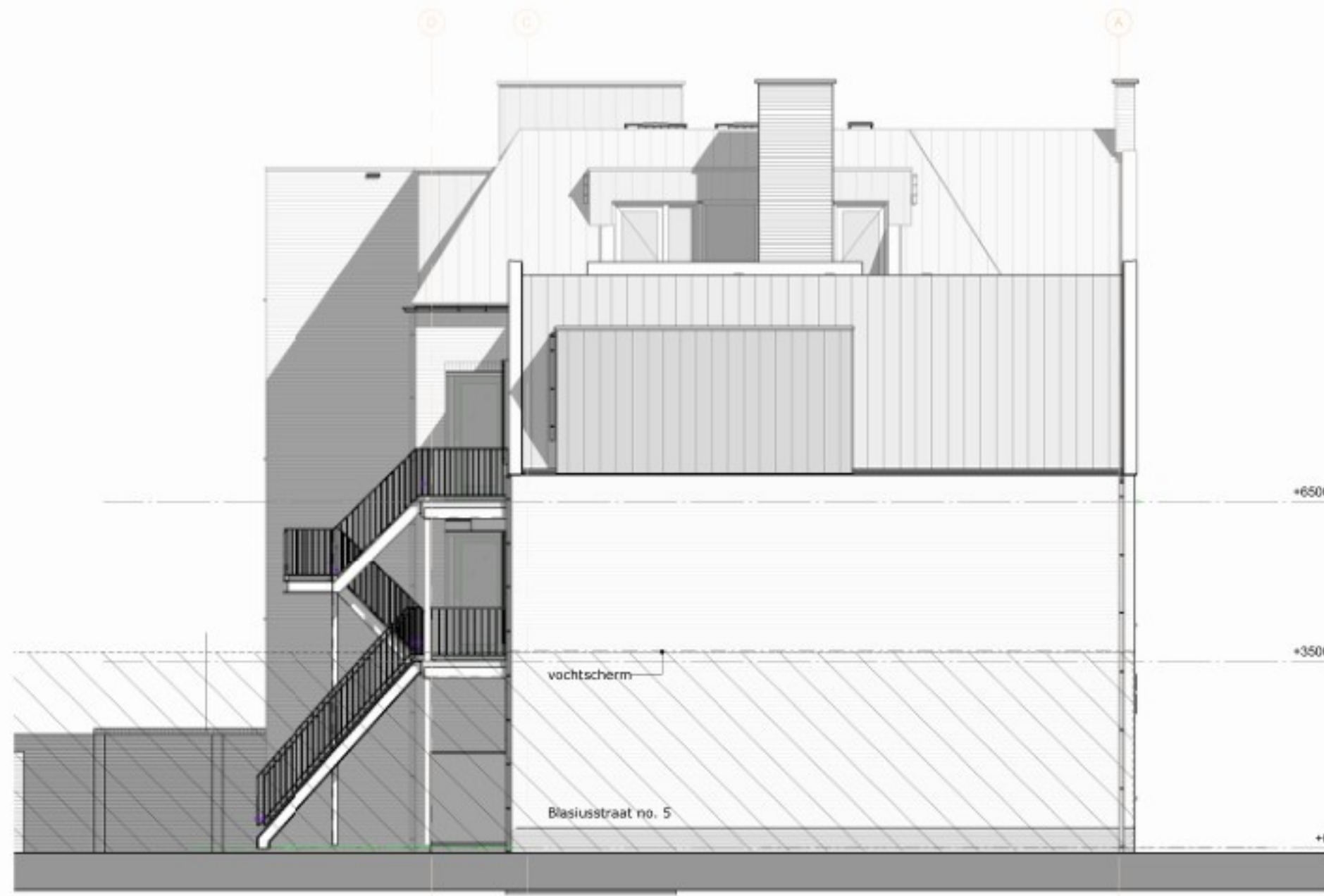
Linkergevel
