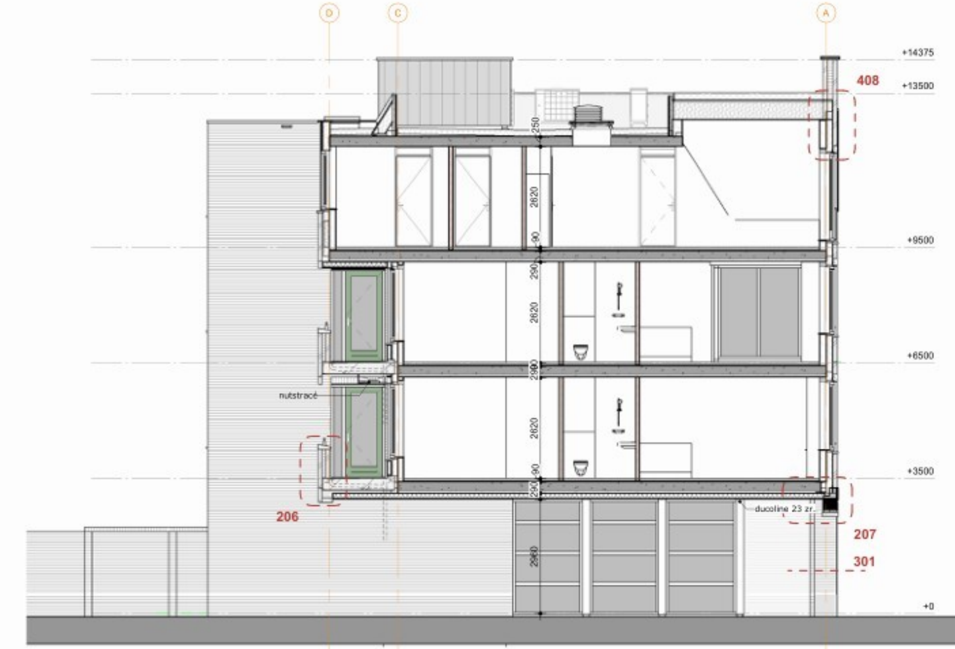
Doorsnede G
