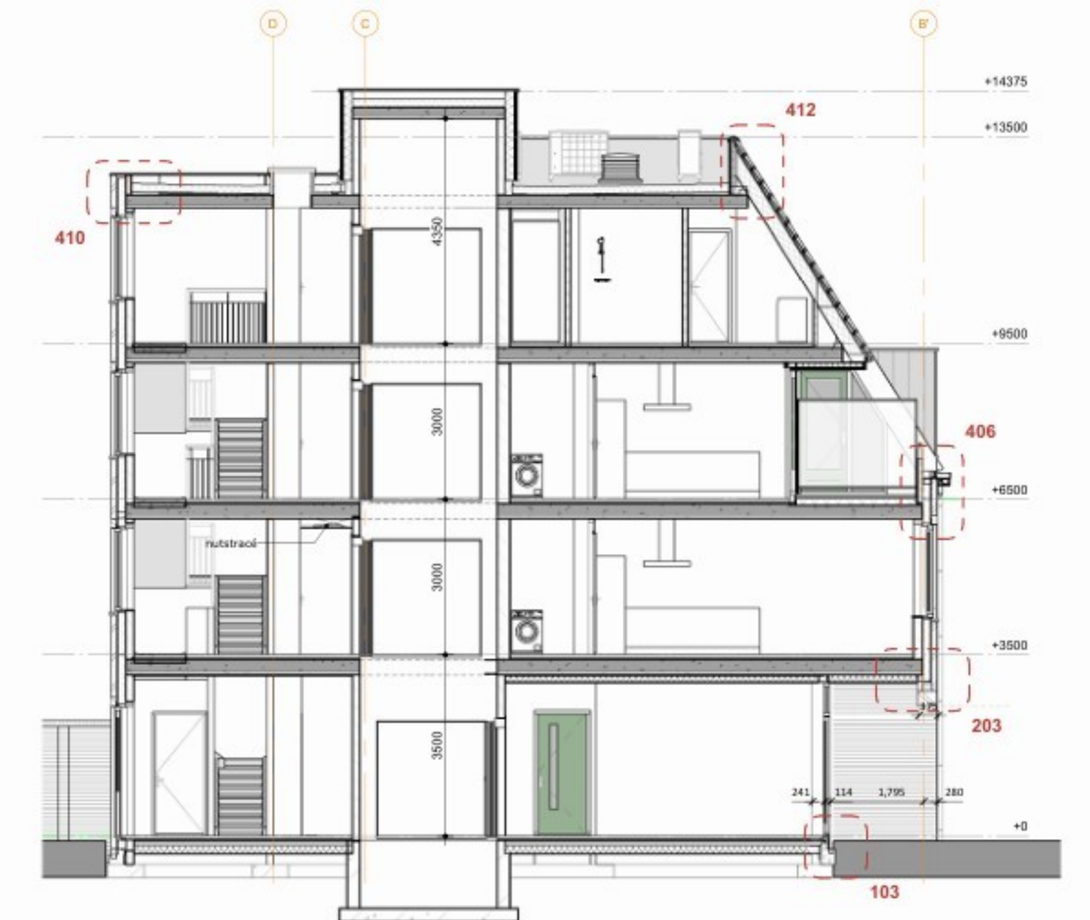
Doorsnede C
