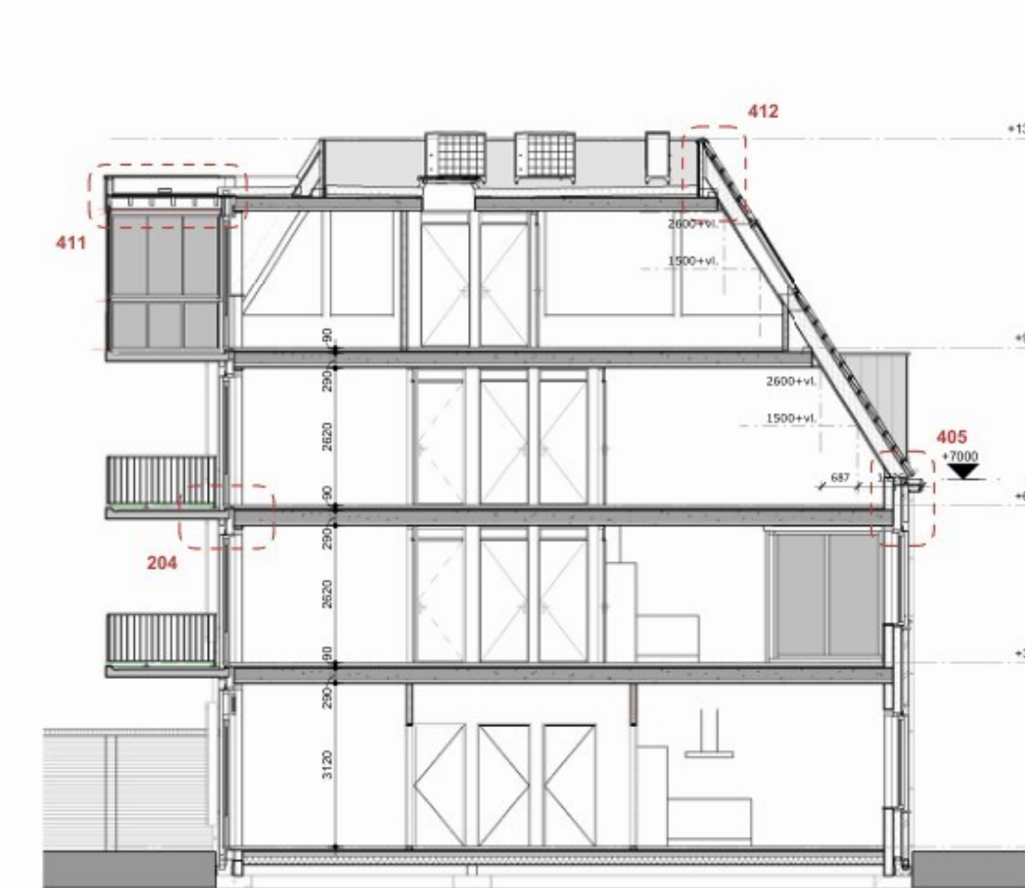
Doorsnede B
