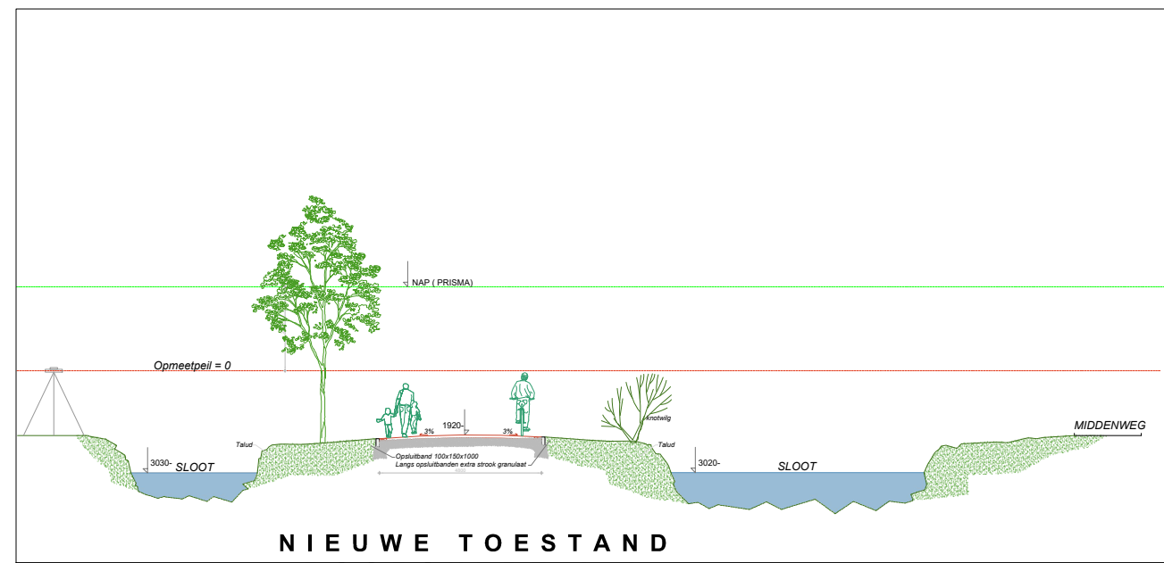
NIEUWE TOESTAND DOORSNED E C-C SCHAAL 1:200
