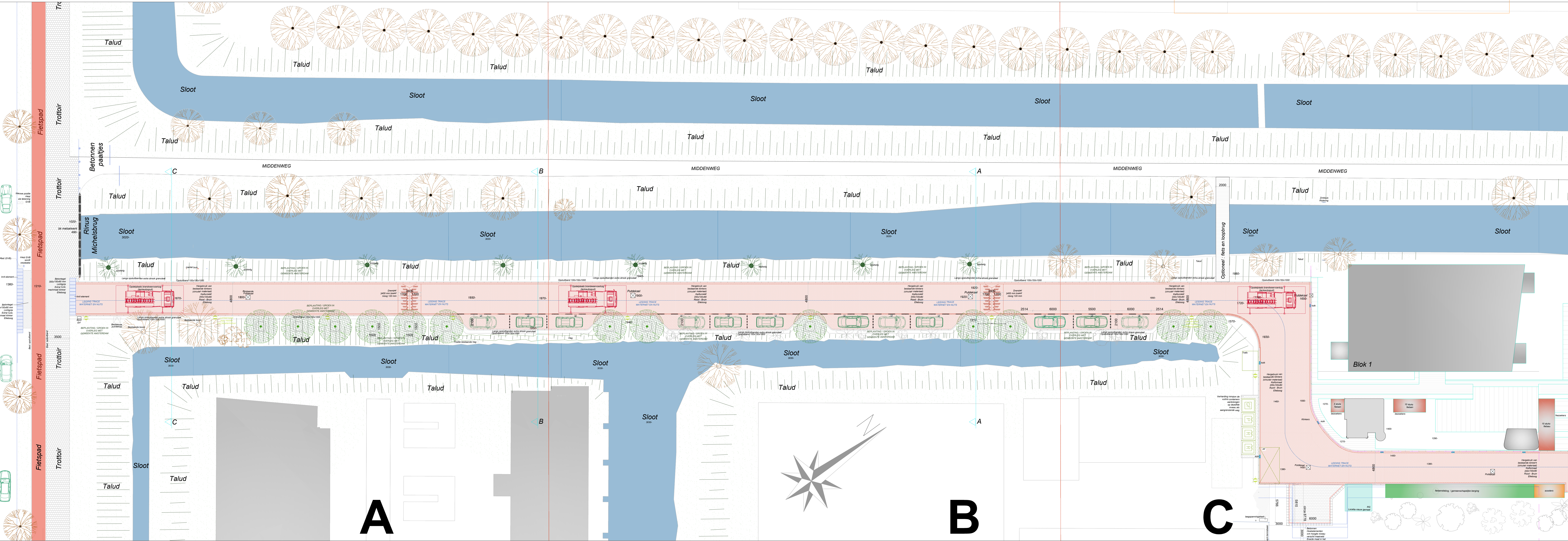
NIEUWE TOESTAND TERREIN SCHAAL 1:200
