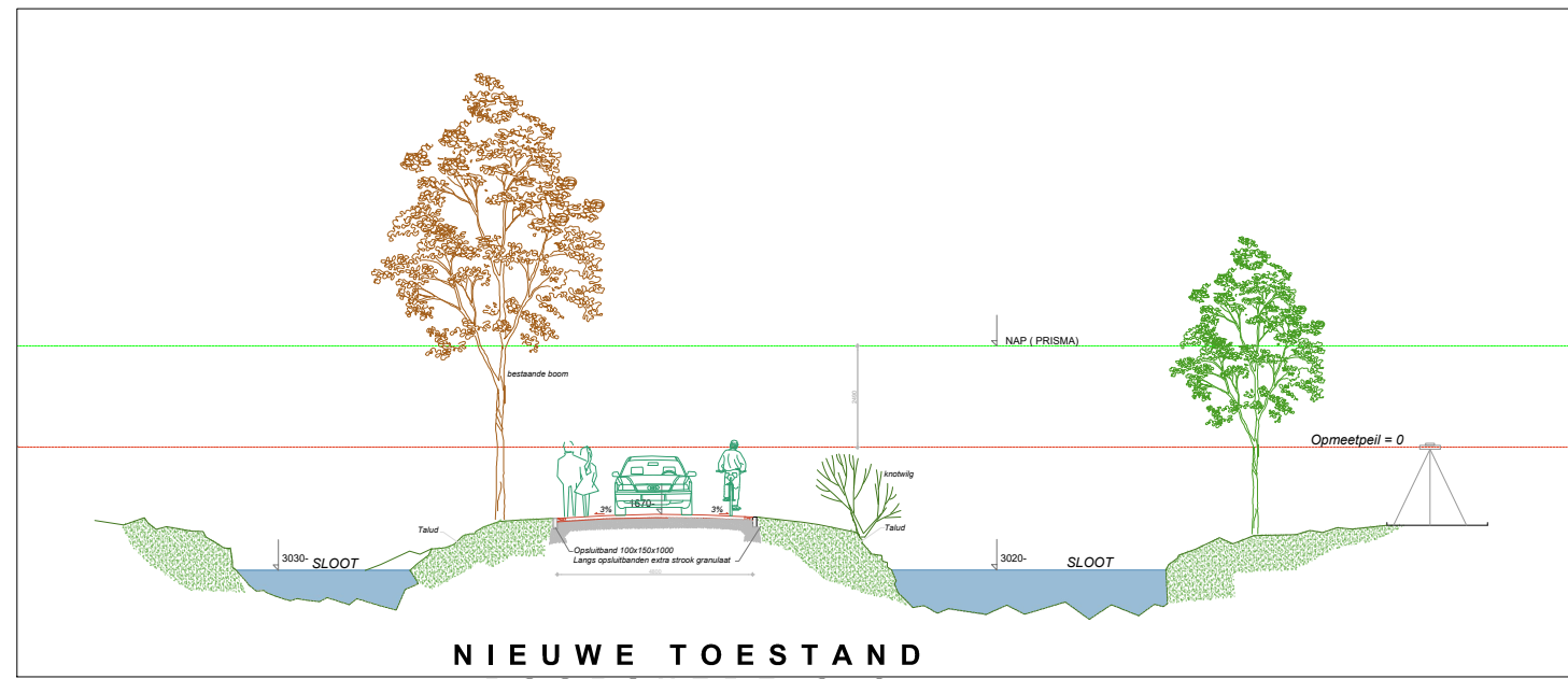
NIEUWE TOESTAND DOORSNED E A-A SCHAAL 1:200
