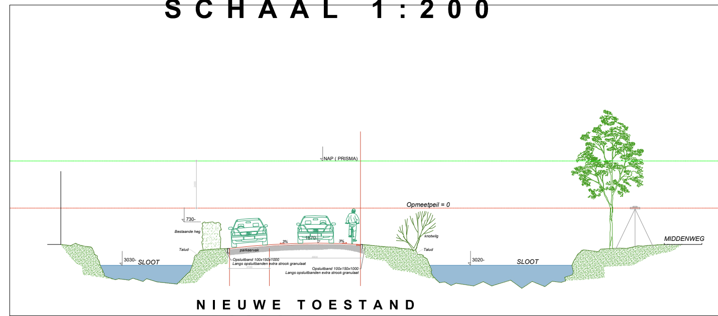
NIEUWE TOESTAND DOORSNED E B-B SCHAAL 1:200
