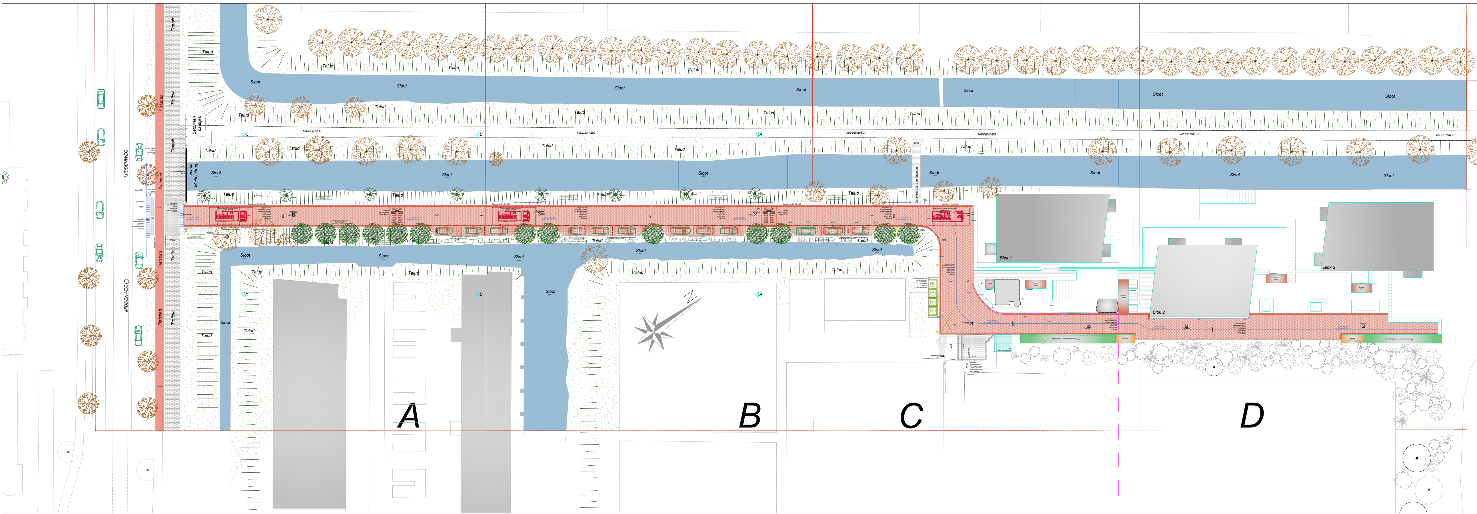
NIEUWE TOESTAND TERREIN SCHAAL 1:500
