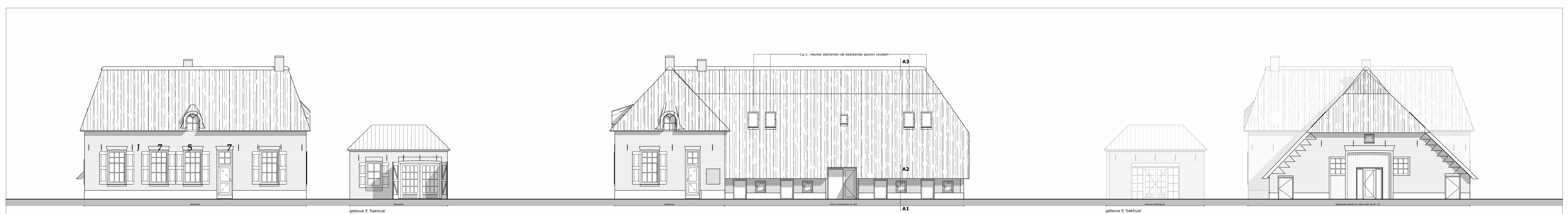
voorgevel rechter zijgevel achtergevel
