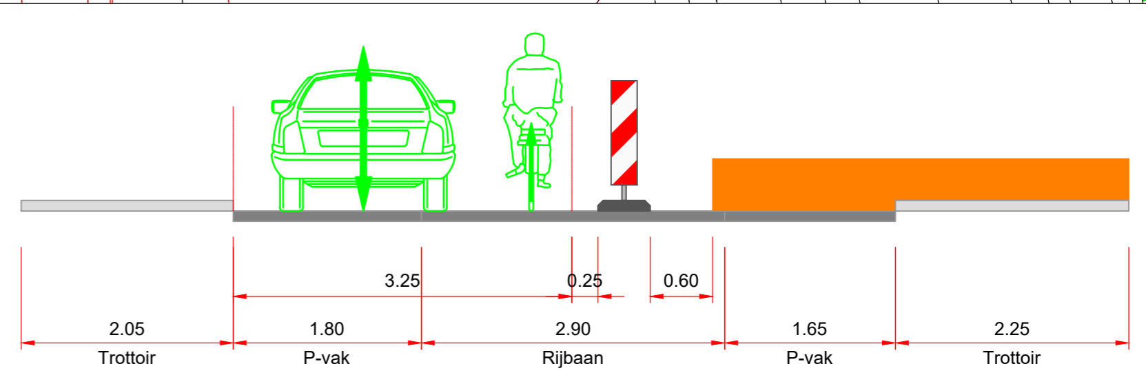
Doorsnede A-A
