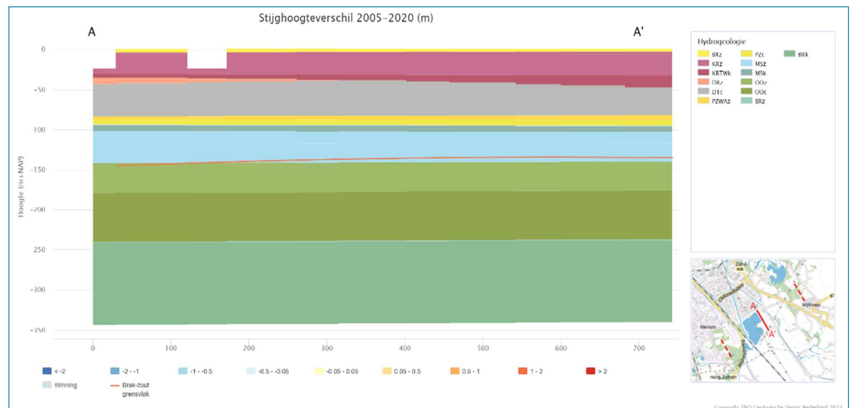
Figuur 2: Geohydrologische bodemopbouw van de onderzoekslocatie (Grondwaterkaart Nederland)
