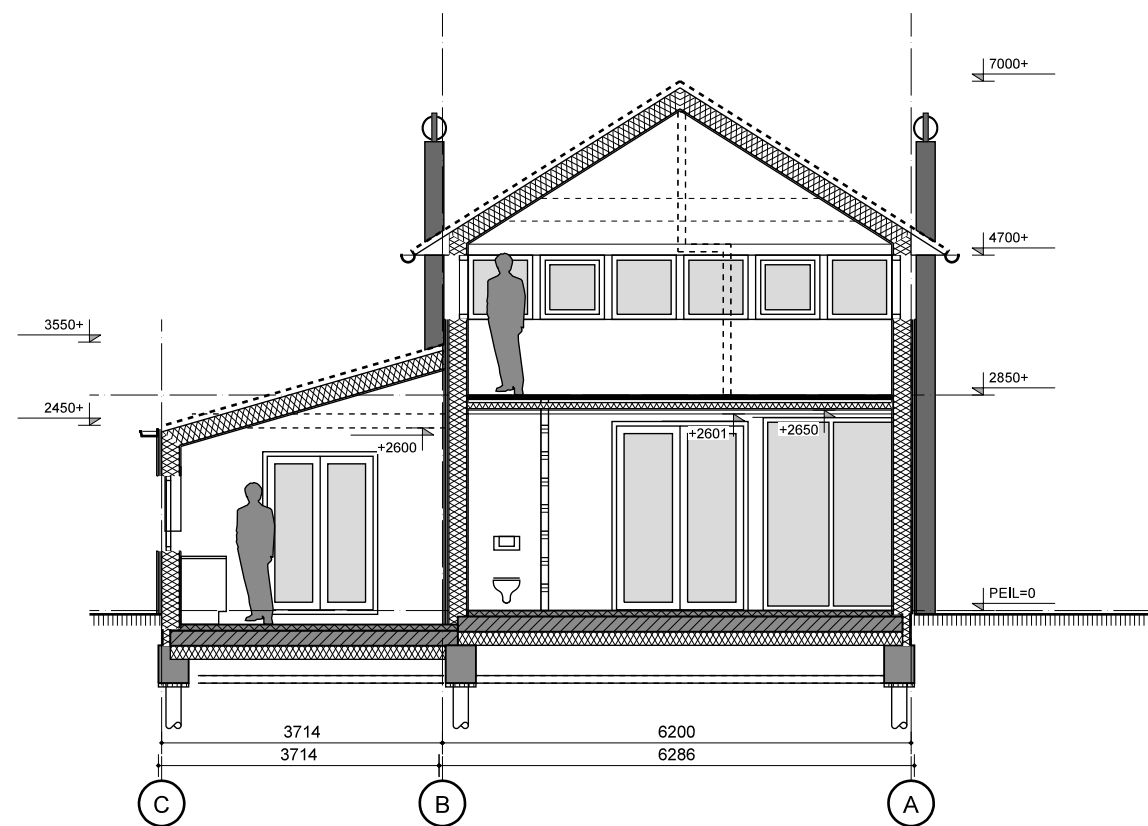
doorsnede A-A
