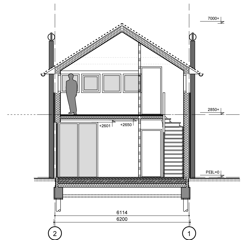
doorsnede B-B
