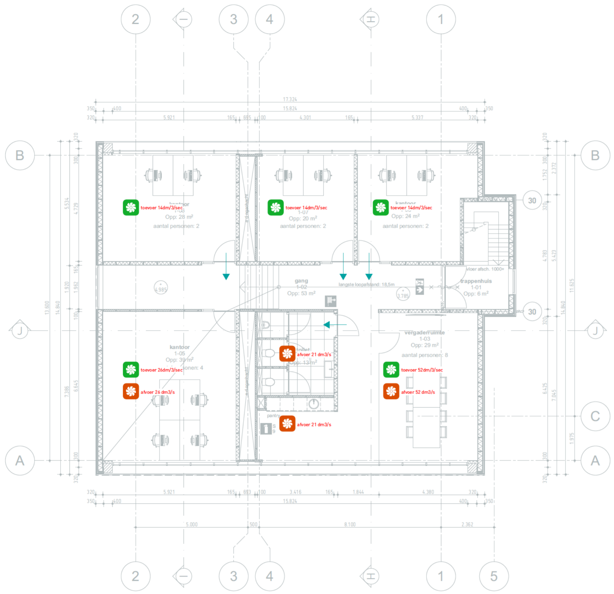
Ventilatie schema: norm: 6,5dm 3 /s/persoon mechanische toe- en afvoer
