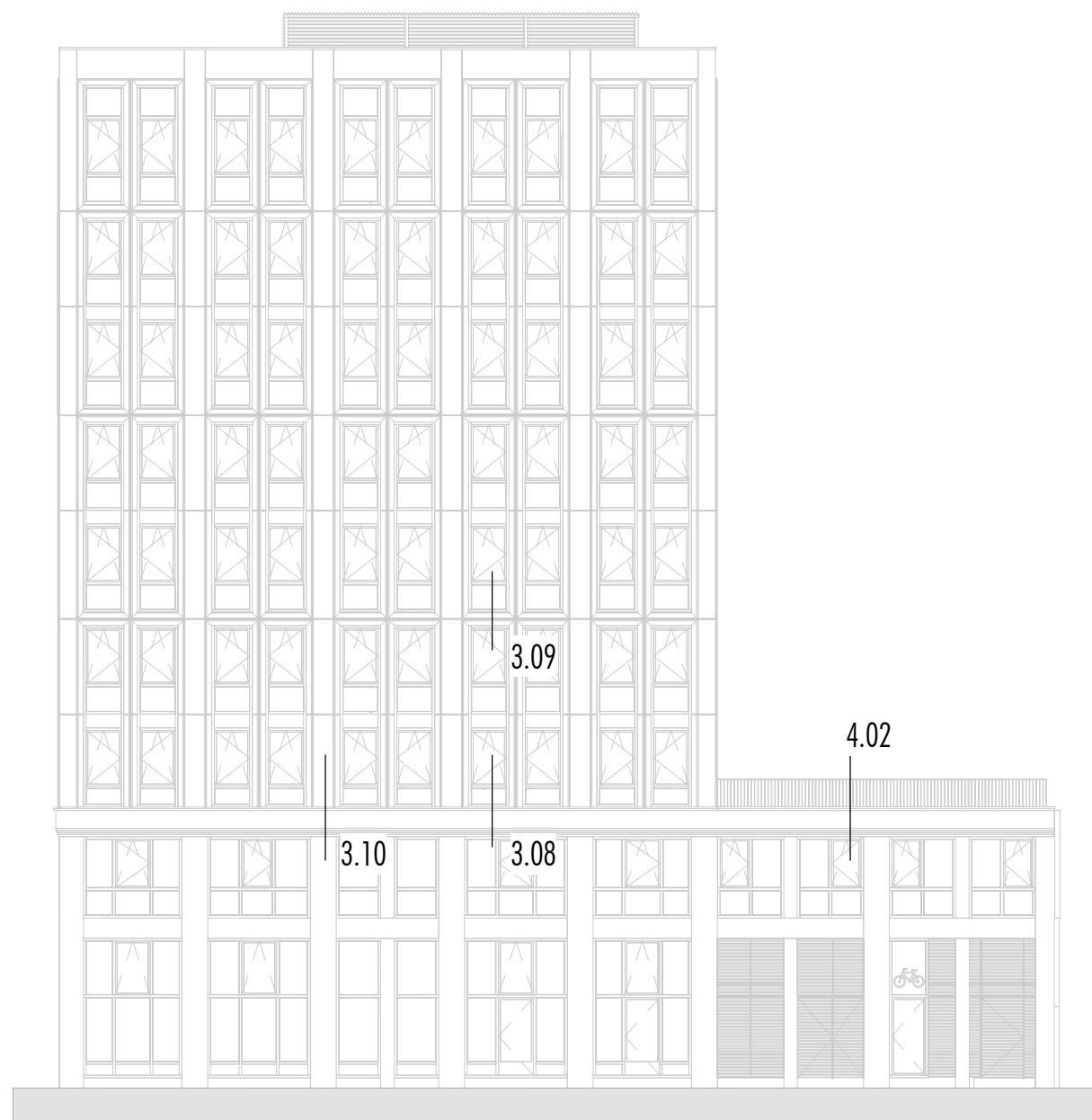
1 WESTGEVEL detailoverzicht schaal 1 : 200
