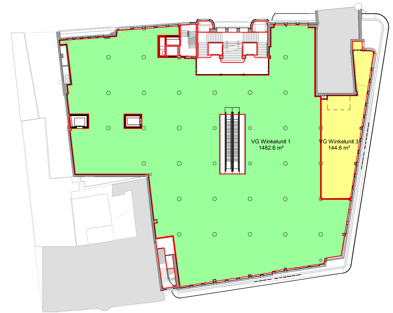
01 eerste verdieping
