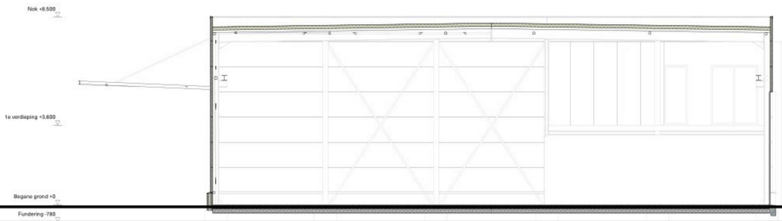
Doorsnede A
