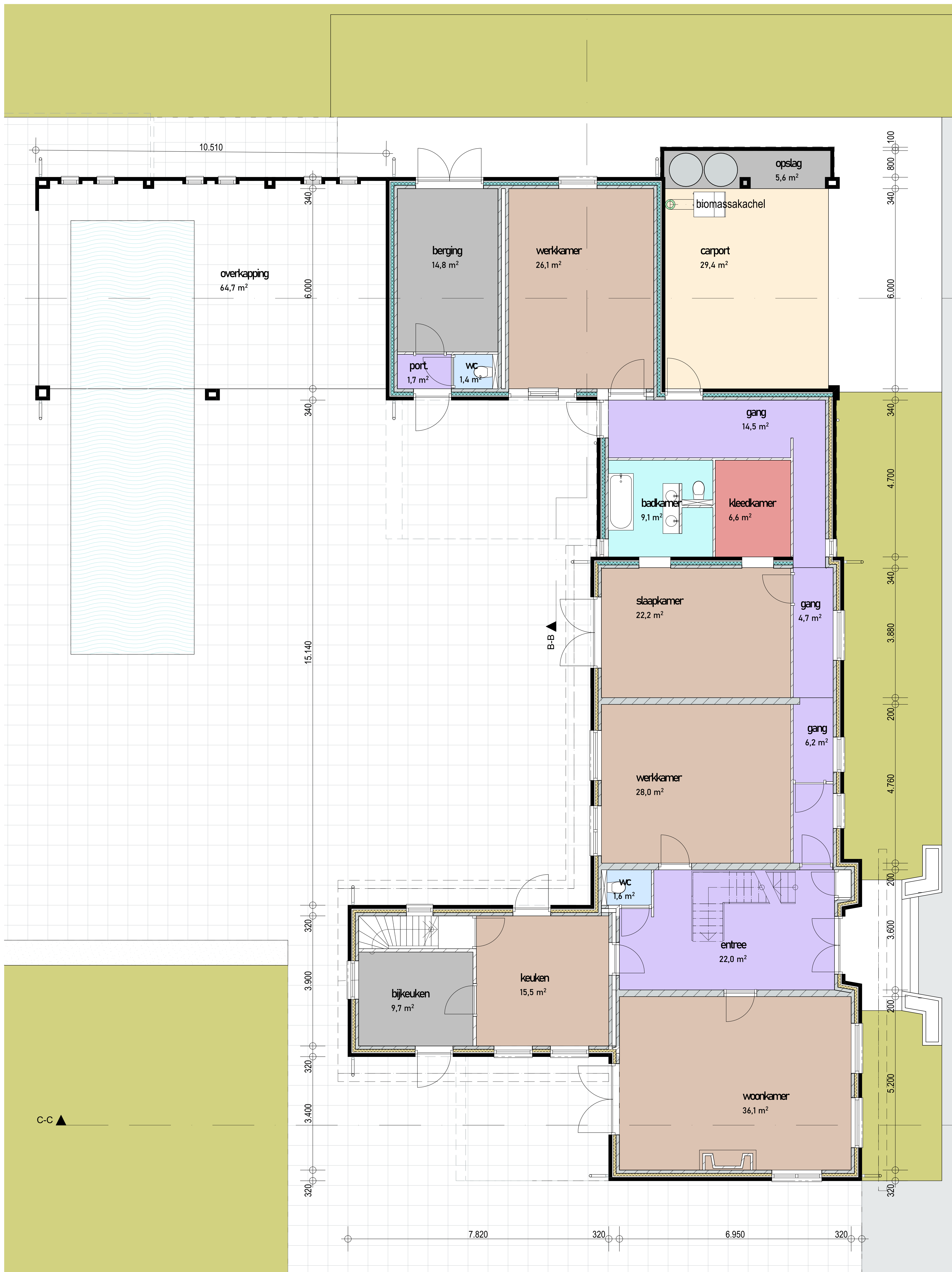
0.1:50 begane grond bestaand
