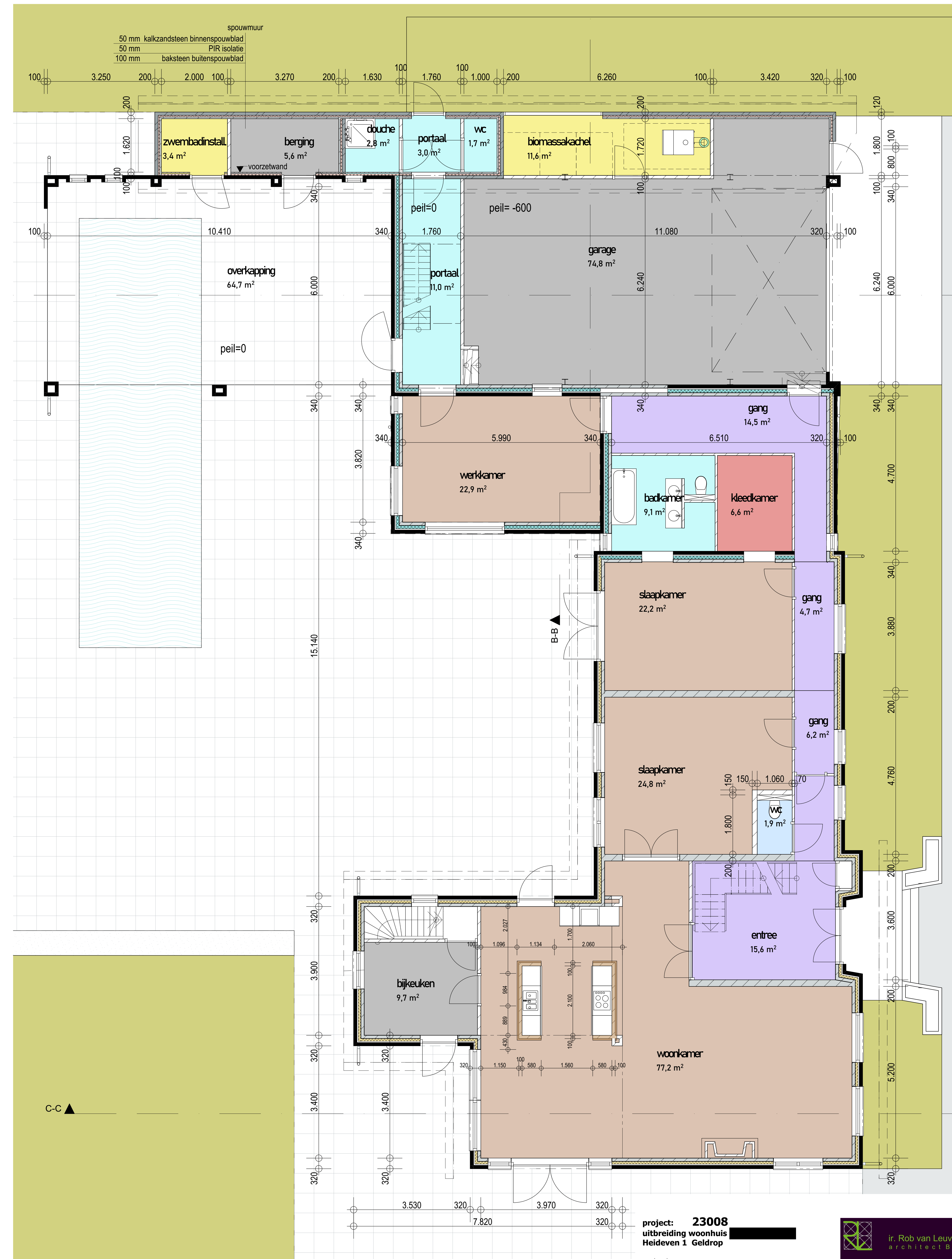
0.2:50 begane grond nieuw
