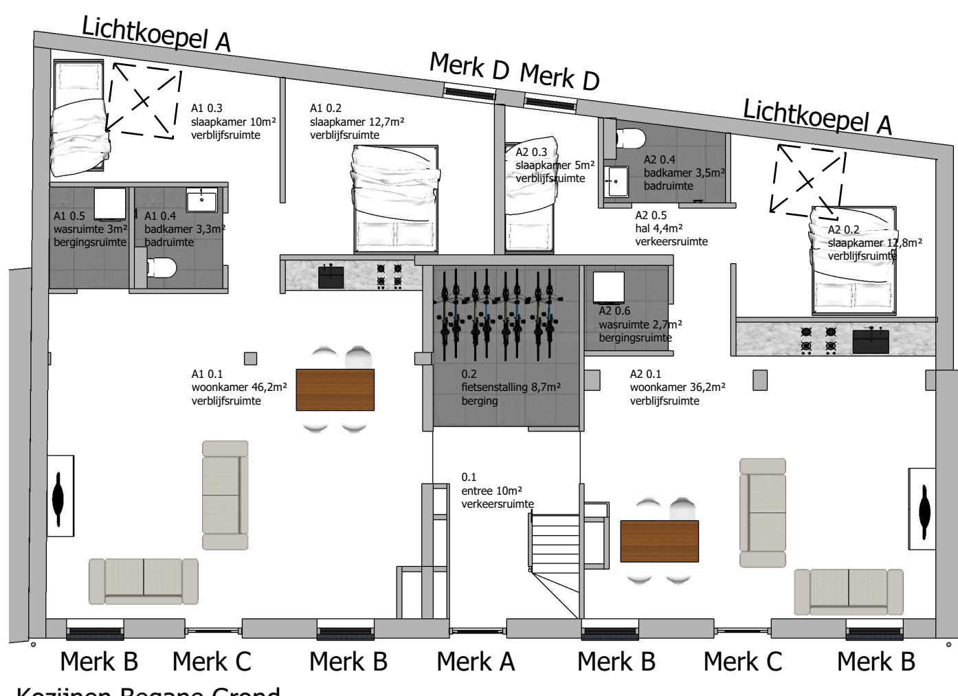
Kozijnen Begane Grond
