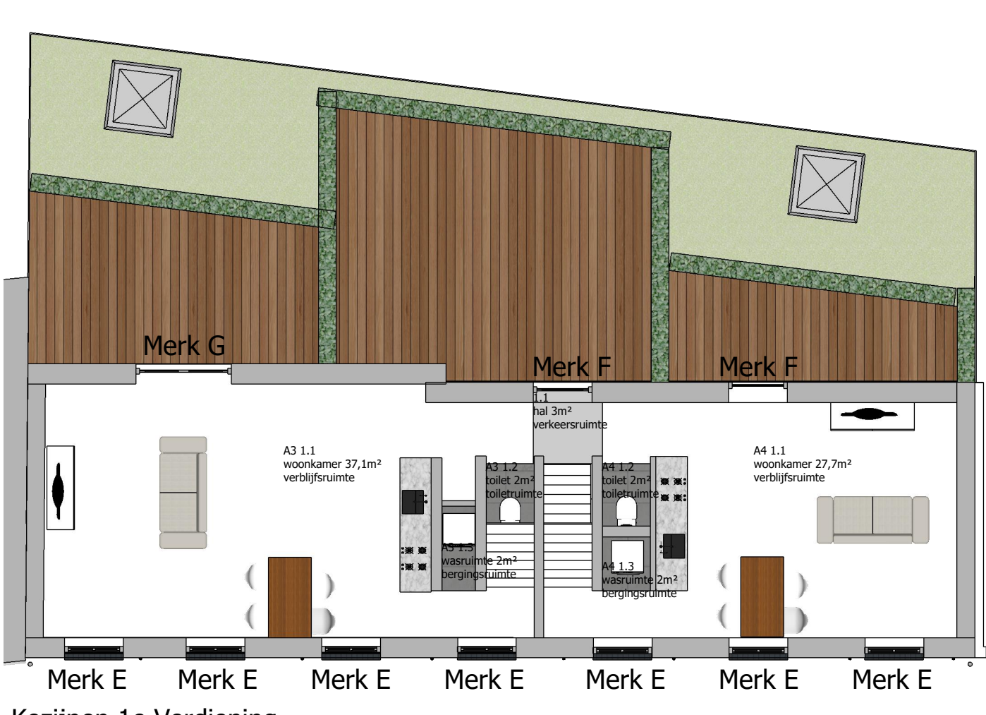
Kozijnen 1e Verdieping
