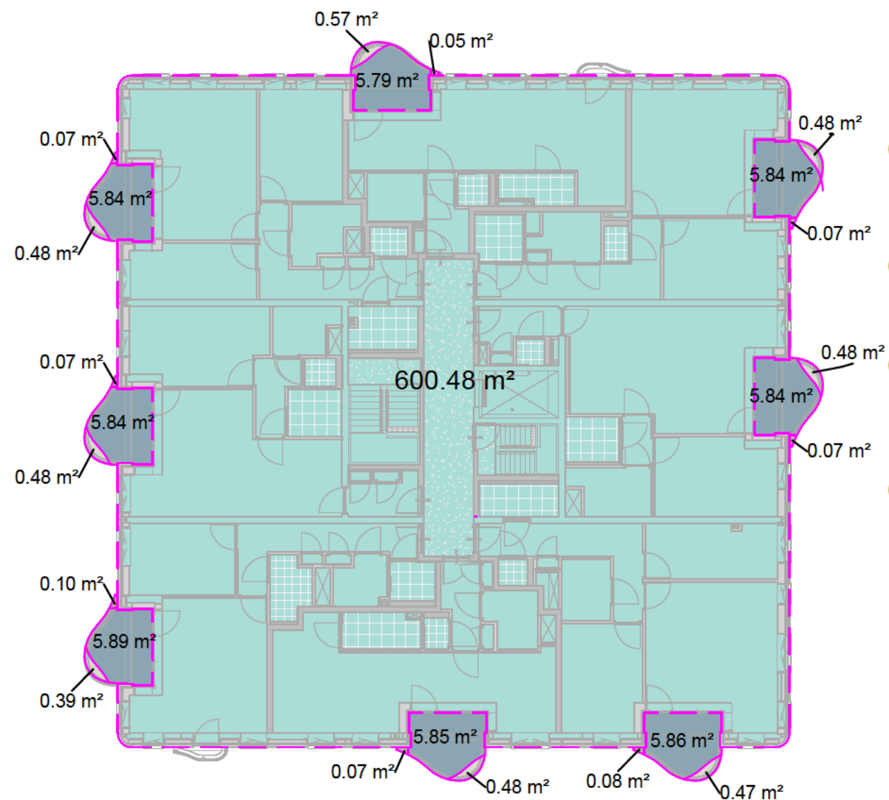
Tweede verdieping P4.1
