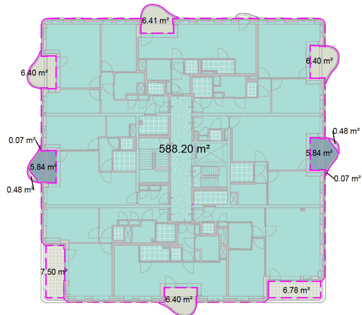
Vierde verdieping P4.1
