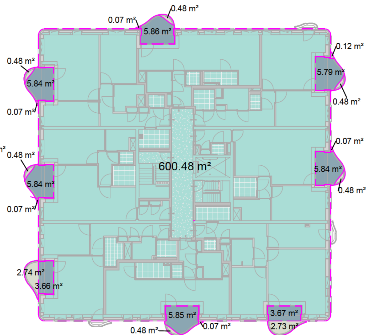
Derde verdieping P4.1
