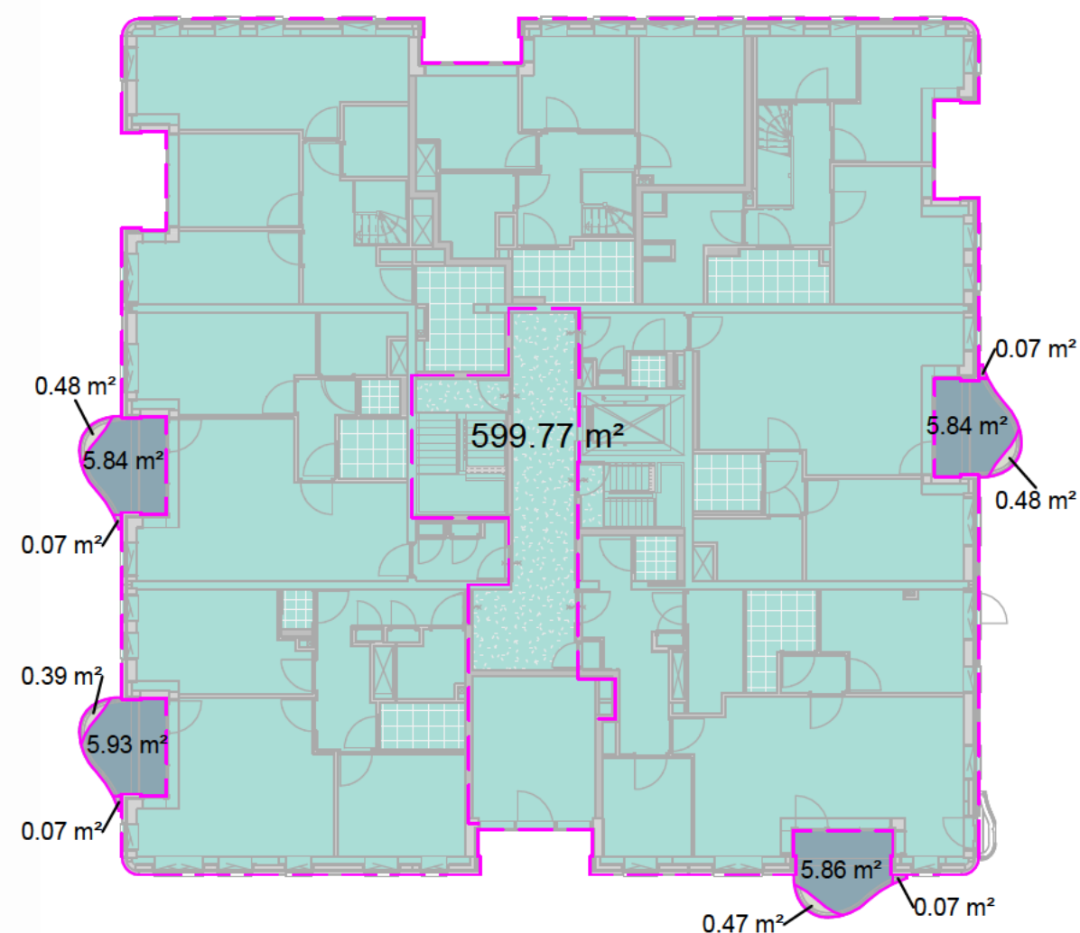
Eerste verdieping P4.1
