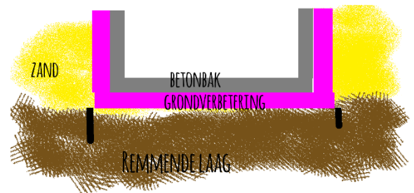
Figuur 8 – principe (paars is maatregel), verticale zwarte strepen is een voorbeeld waarbij restant damwand (beneden onderkant barrière) niet verwijderd wordt
