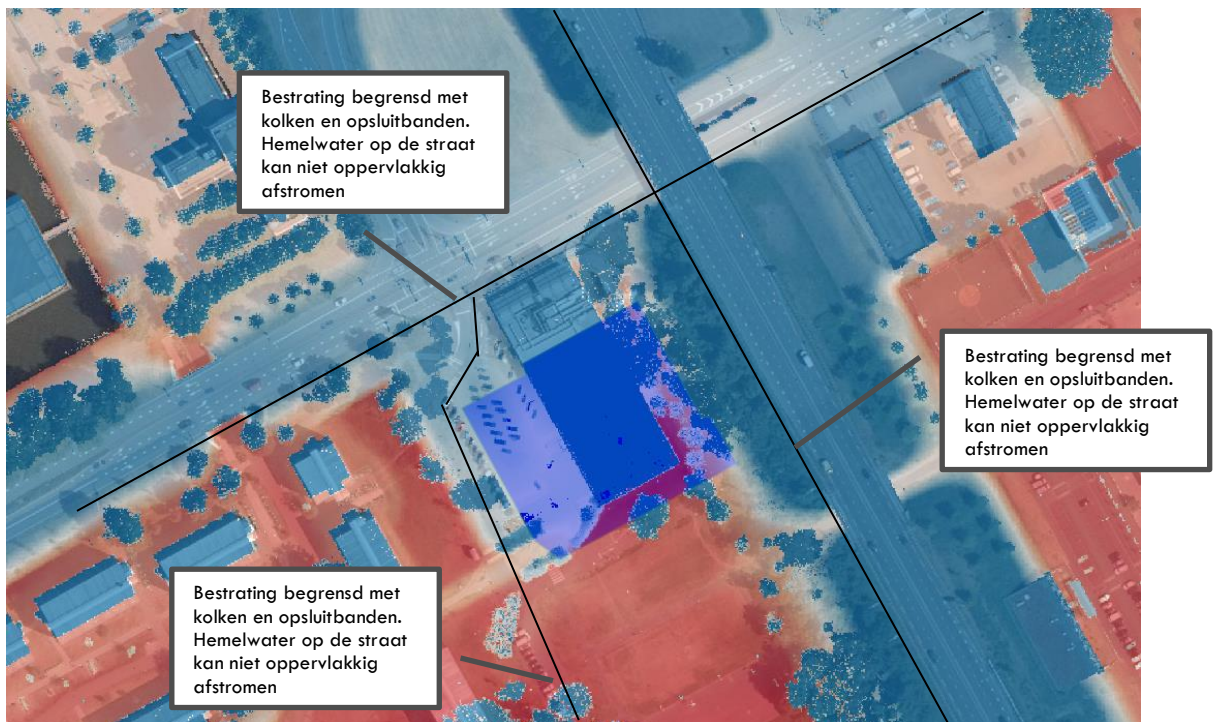
Figuur 7 - maaiveldhoogte effect (rood=laag maaiveld en blauw=hoog maaiveld)
