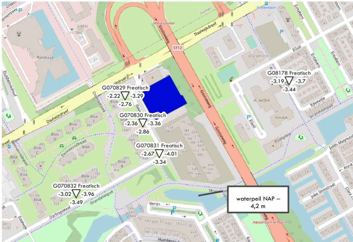
Figuur 6 – grondwaterstanden ten opzichte van NAP [m] (boven driehoek=peilbuis naam, onder driehoek=gemiddelde grondwaterstand, links driehoek=maatgevend hoge grondwaterstand, rechts driehoek=maatgevende lage grondwaterstand)
