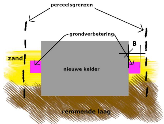
Figuur 12 – principe (paars is maatregel)
