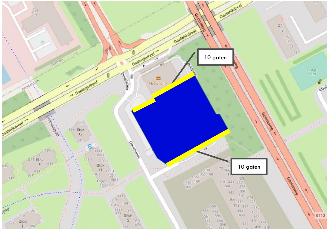
Figuur 13 – souterrain is grondwaterneutraal bij toepassen maatregelen langs gevels welke geel zijn (voor alle oplosrichtingen).
