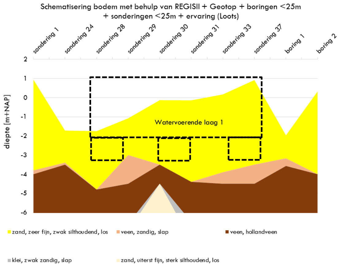
Figuur 4 – schematisering bodem
