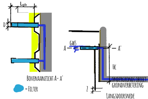
Figuur 11 - principe (blauw is maatregel)
