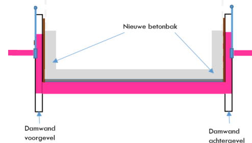
Figuur 9 – principe (paars is maatregel)
