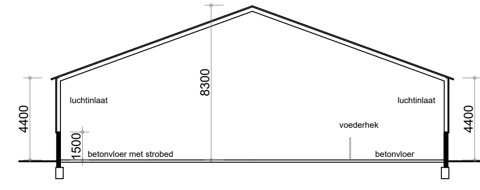
- Doorsnede D - D gebouw 4 -
