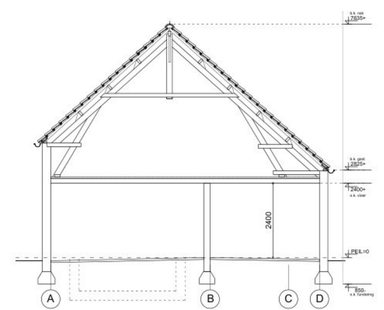
Doorsnede A
