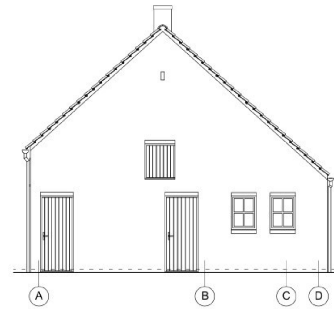
Rechter zijgevel
