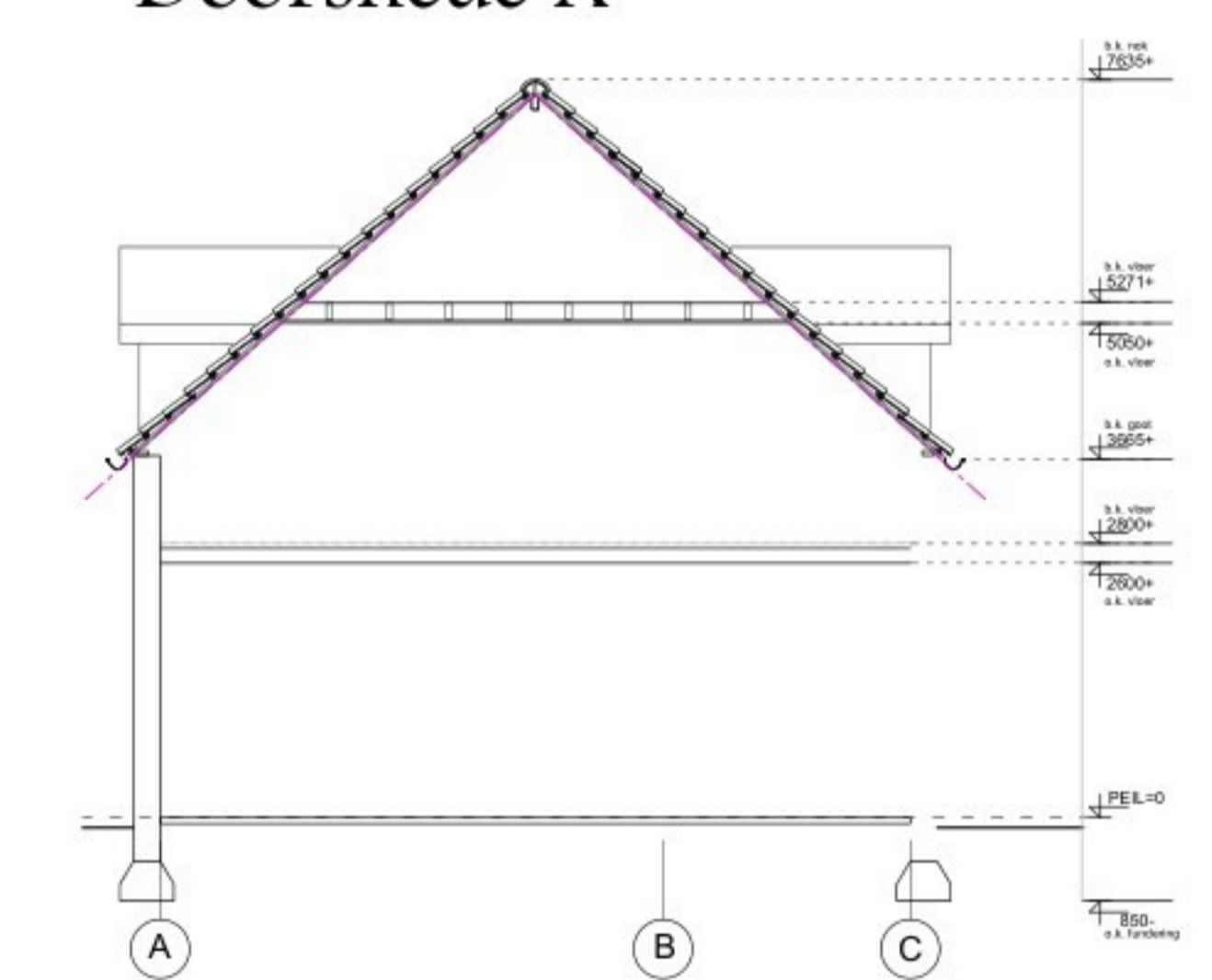
Doorsnede B
