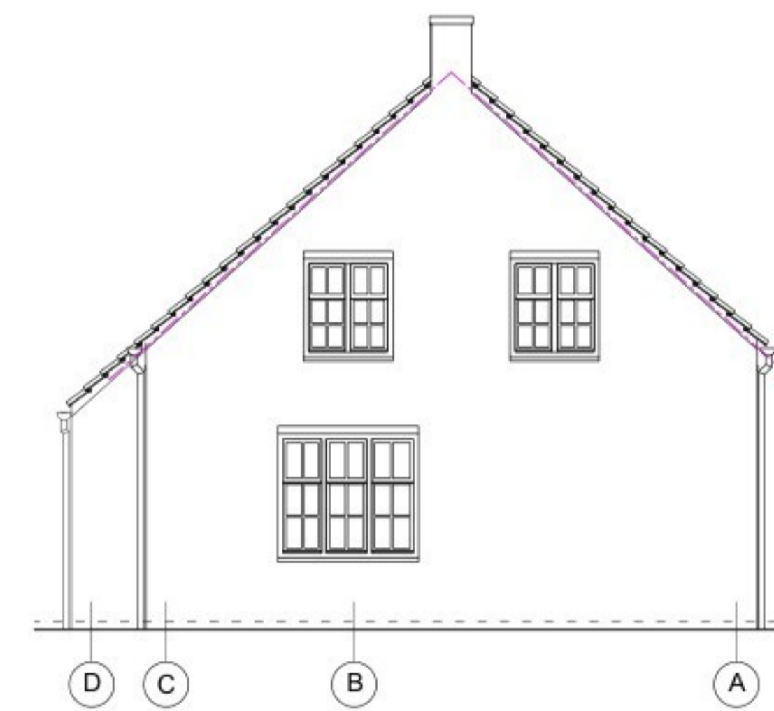
Linker zijgevel
