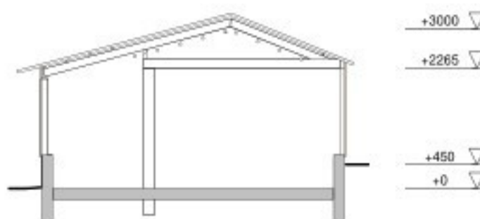
Bestaande doorsnede AB 1 : 100
