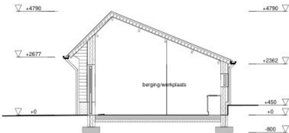
Nieuwe doorsnede A-A 1 : 100
