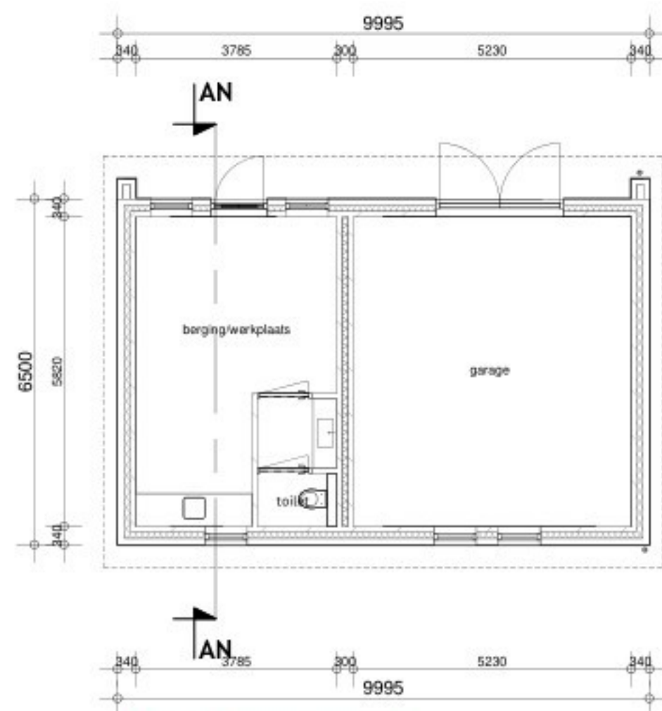
Nieuwe begane grond 1 : 100
