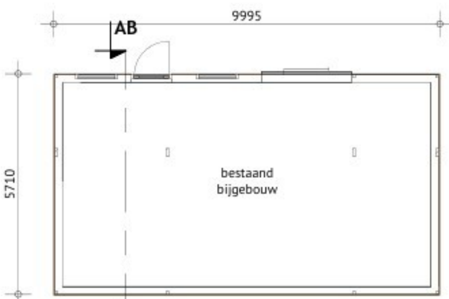
Bestaande begane grond 1 : 100
