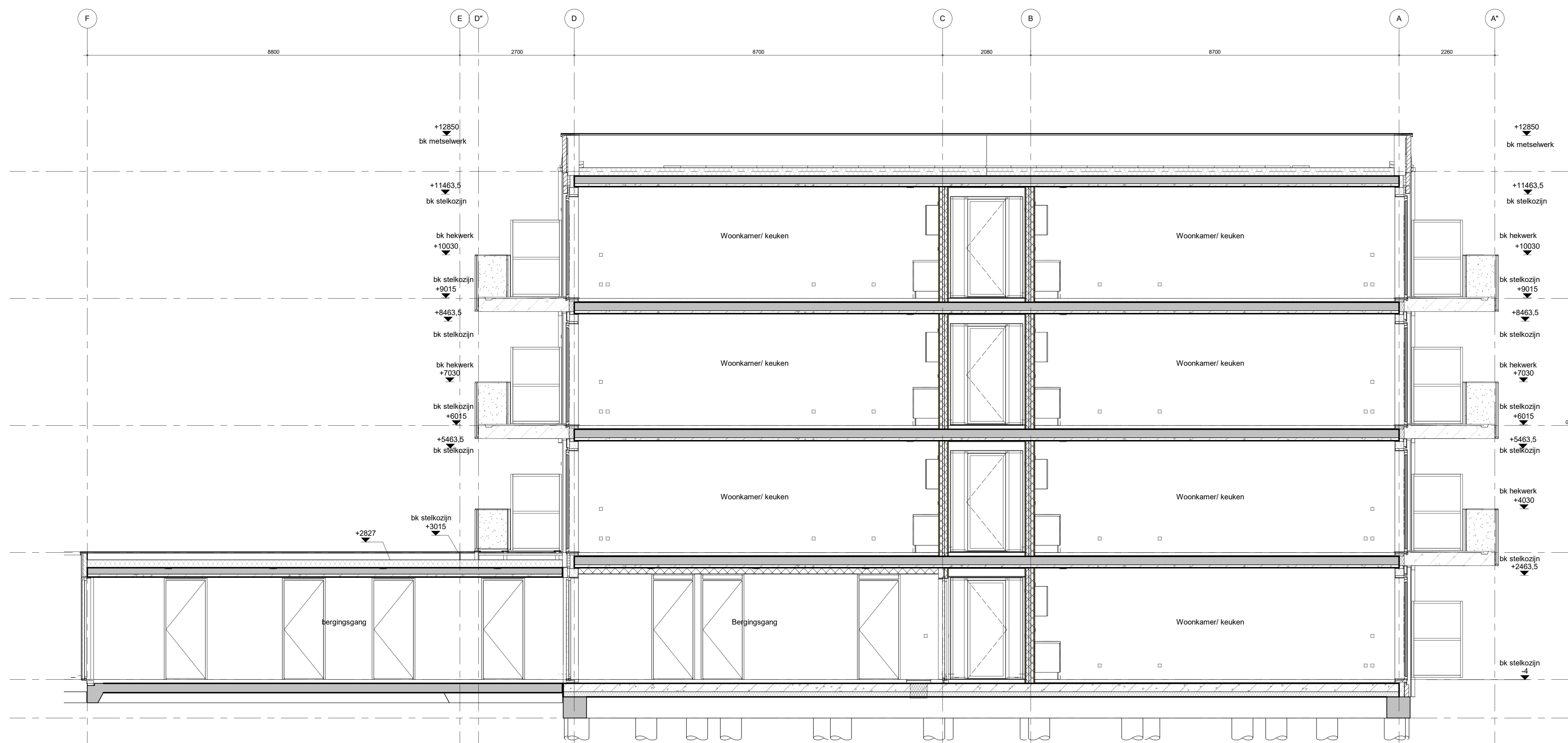
doorsnede tussen as-07/as-08 1:50
