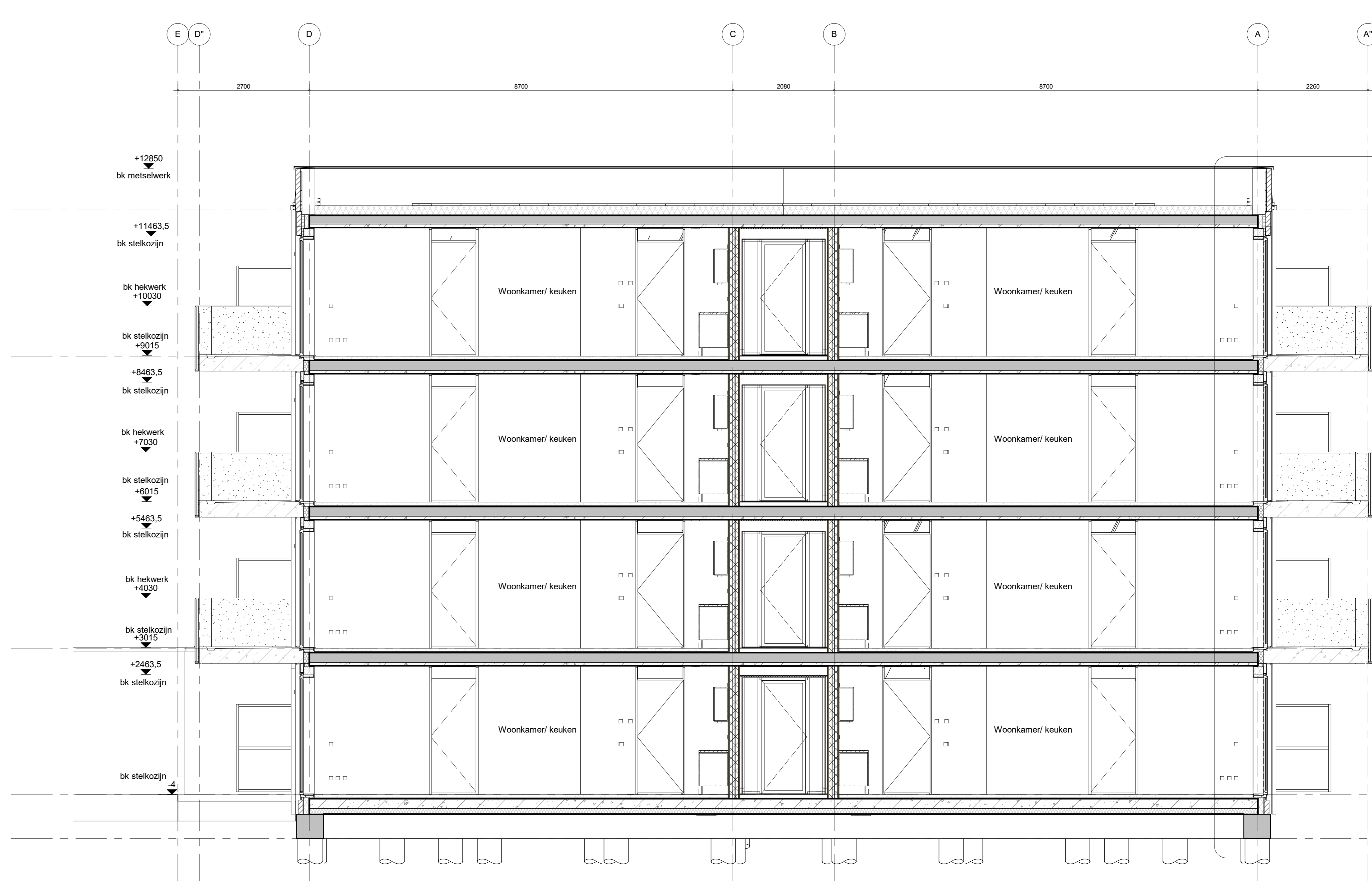
doorsnede tussen as-08/as-09 1:50
