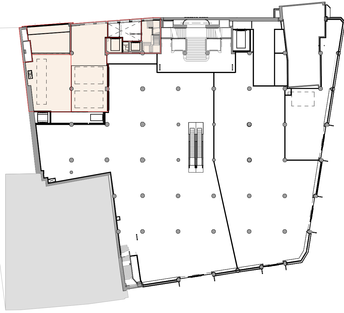
00a tussenverdieping
