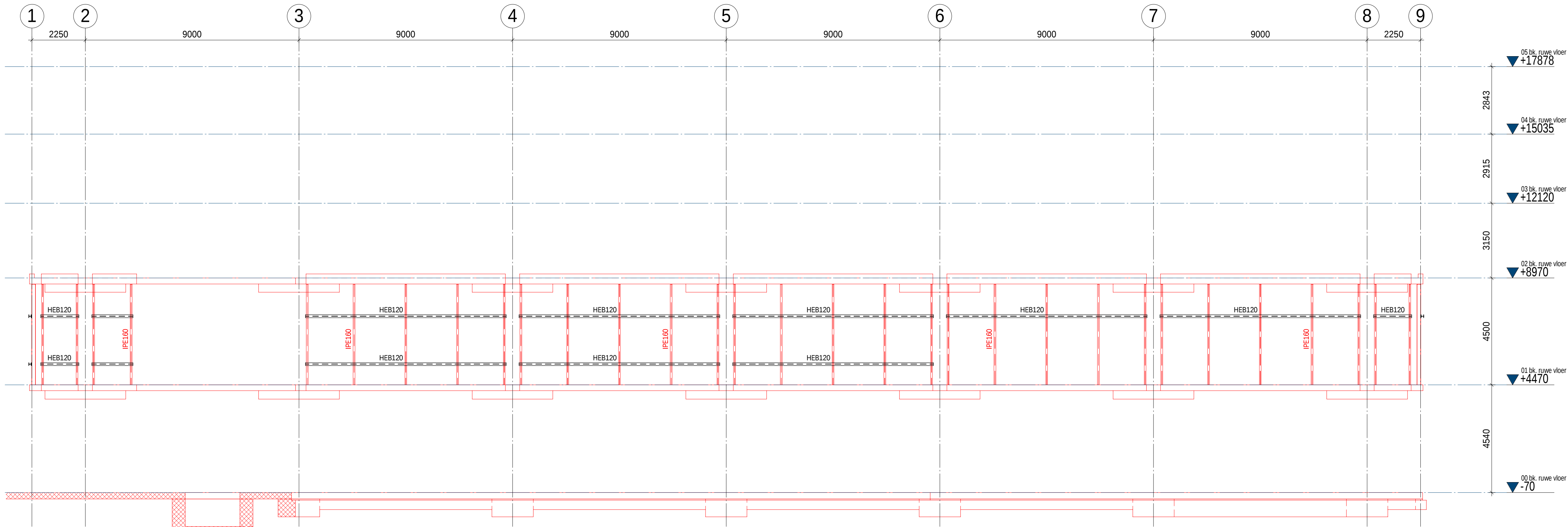
Aanzicht as A 1 : 100
