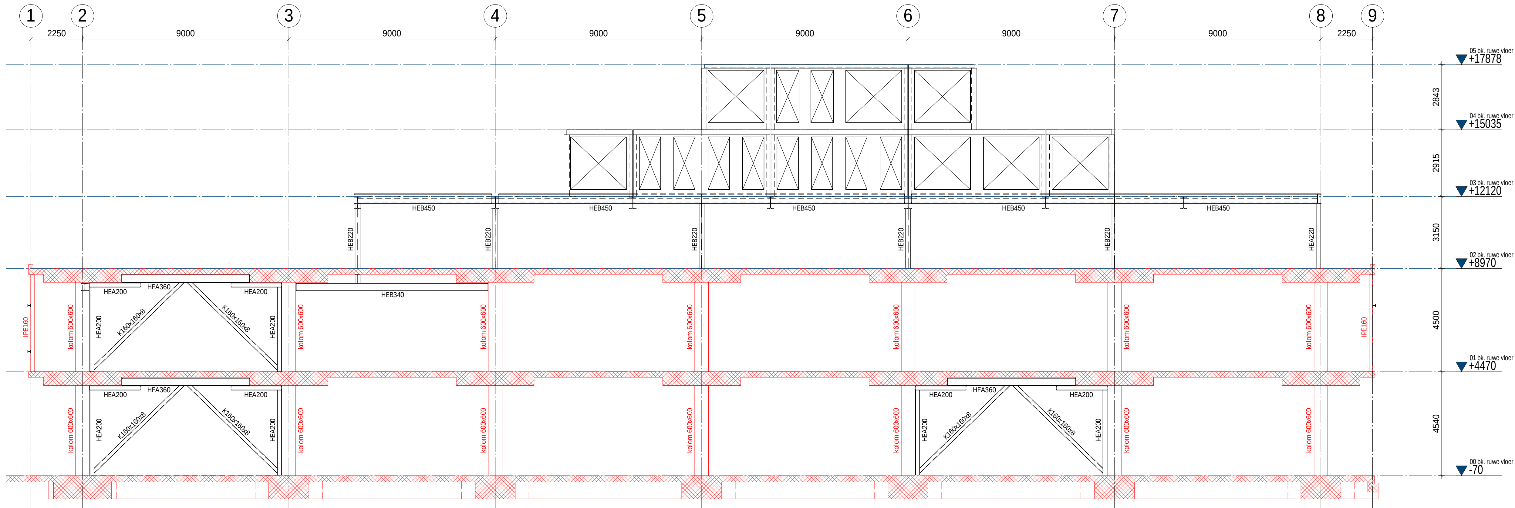
Aanzicht as B 1 : 100
