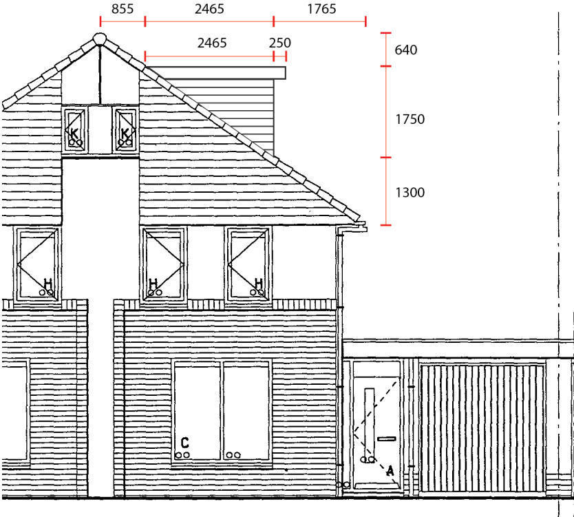
Vooraanzicht (1:100)
