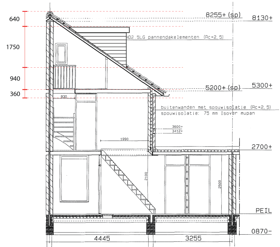
Voorgevel aanzicht doorsnede (1:100)
