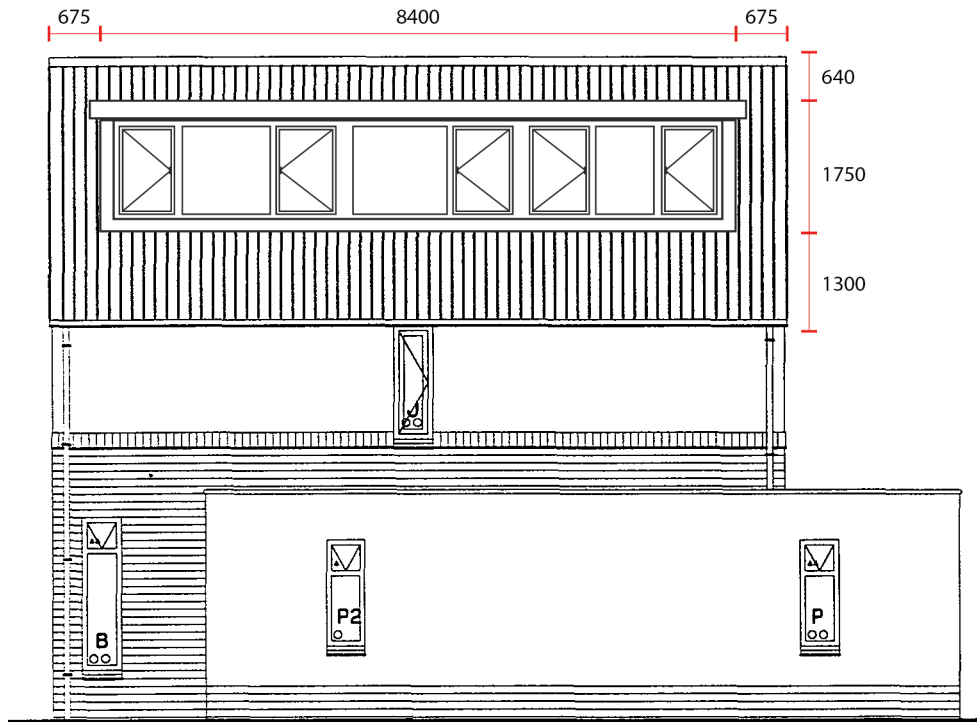
Zijaanzicht (1:100)
