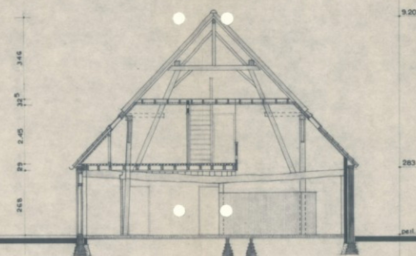
DOORSNEDE B-B
