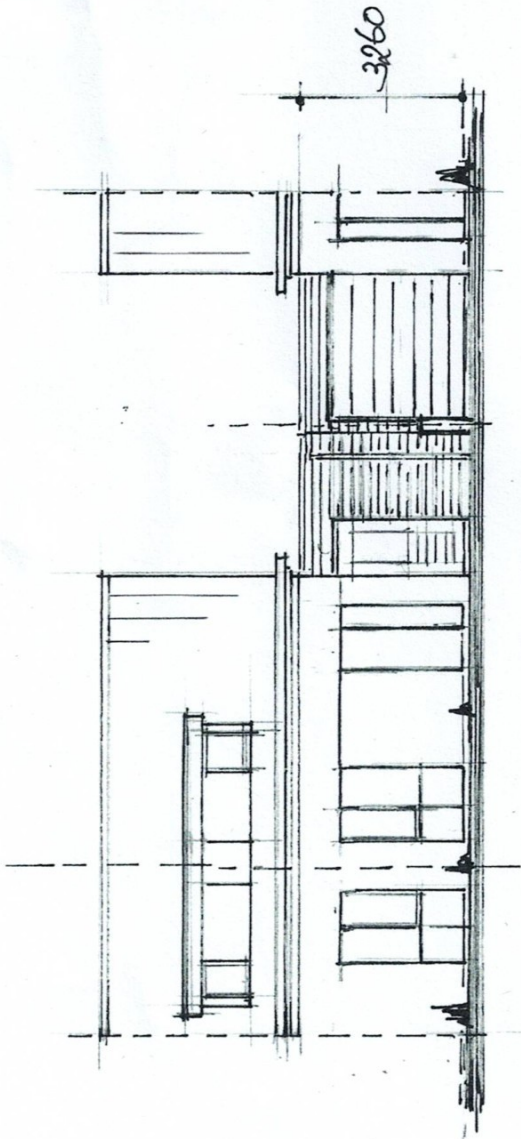
voorgevel. oud.
